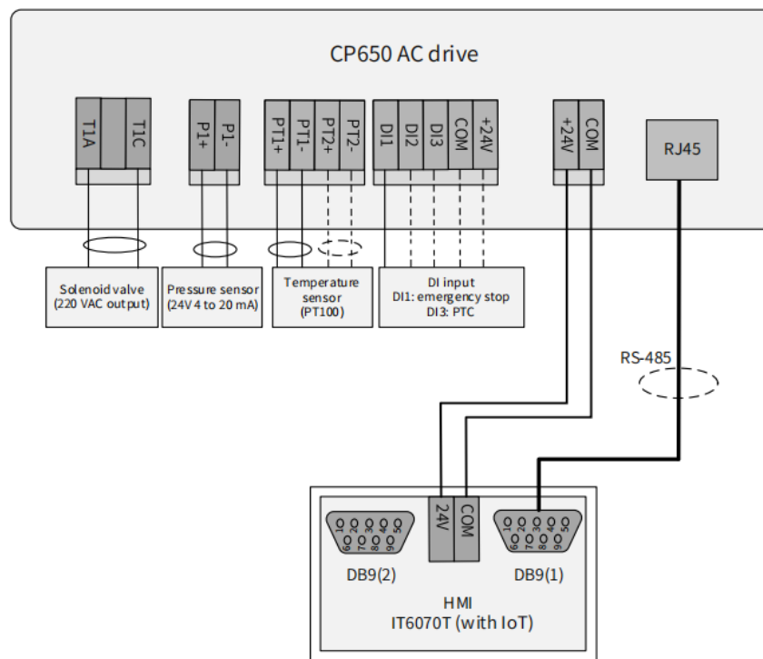
Kuva 2-9 Ohjauspäätejohdotus
